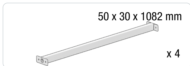
E Verbindungsstrebe | Connecting strut | Entretoise de connexion
