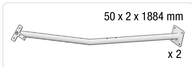
G Kleiner Ständer | Small stand | Petite supports
